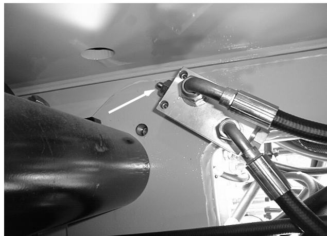
Figure 2-5. Contacteur de fin de course verticale de la flèche de tourelle
