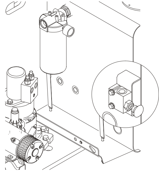
Figure 4-7. Vanne de remise à niveau
