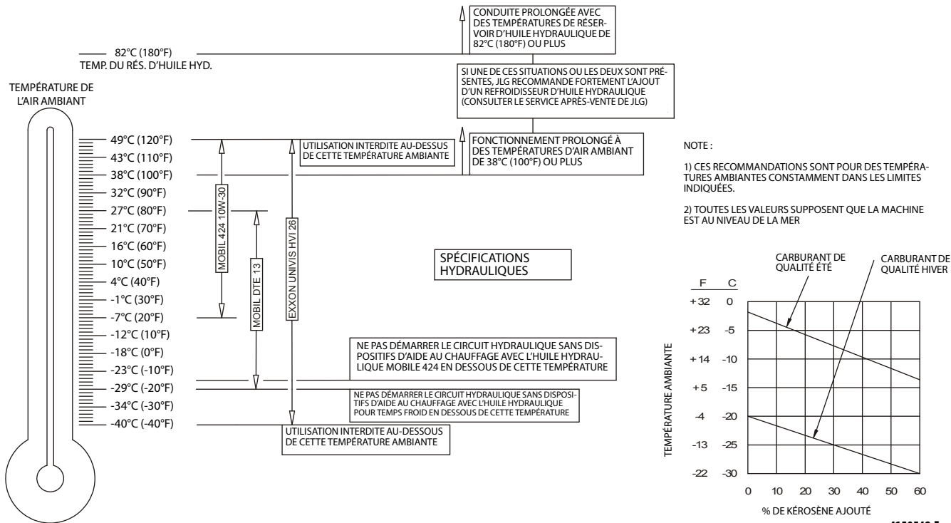
Figure 6-2. Spécifications de température de fonctionnement du moteur — Deutz — Fiche 2 sur 2
