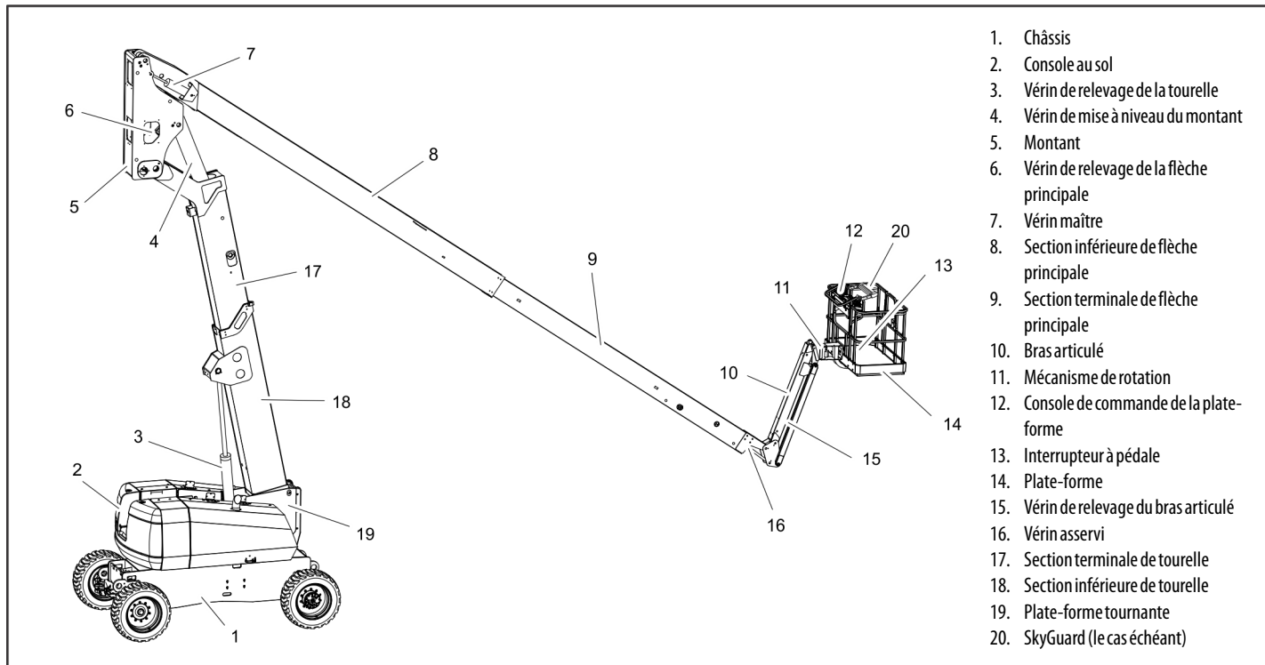
Figure 2-1. Nomenclature de base
