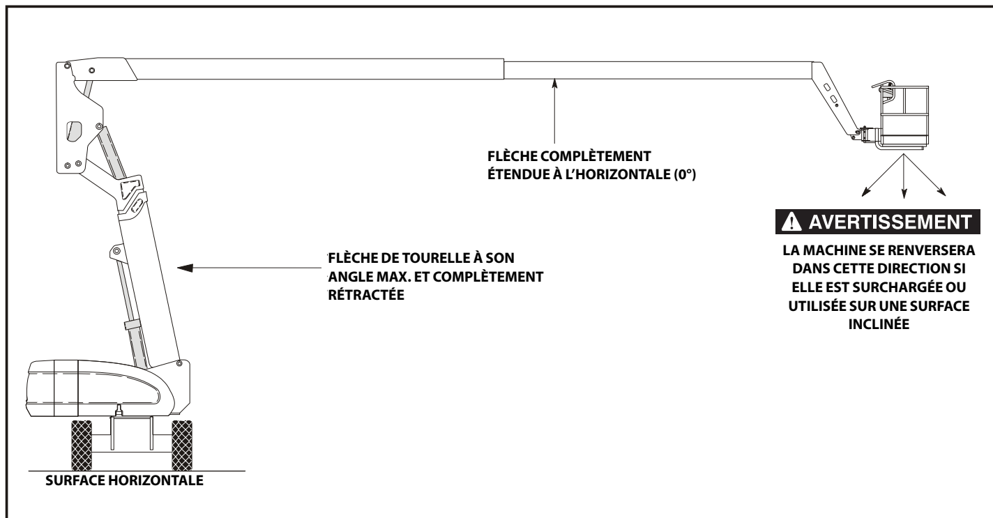
Figure 4-1. Position la moins stable vers l'avant
