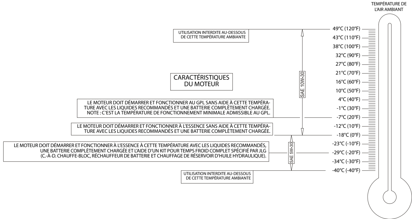
Figure 6-3. Spécifications de température de fonctionnement du moteur — GM — Fiche 1 sur 2
