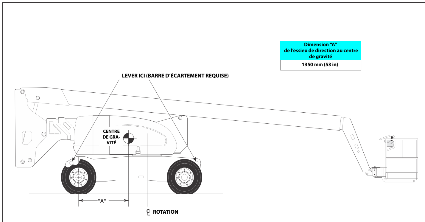
Figure 4-5. Tableau de levage
