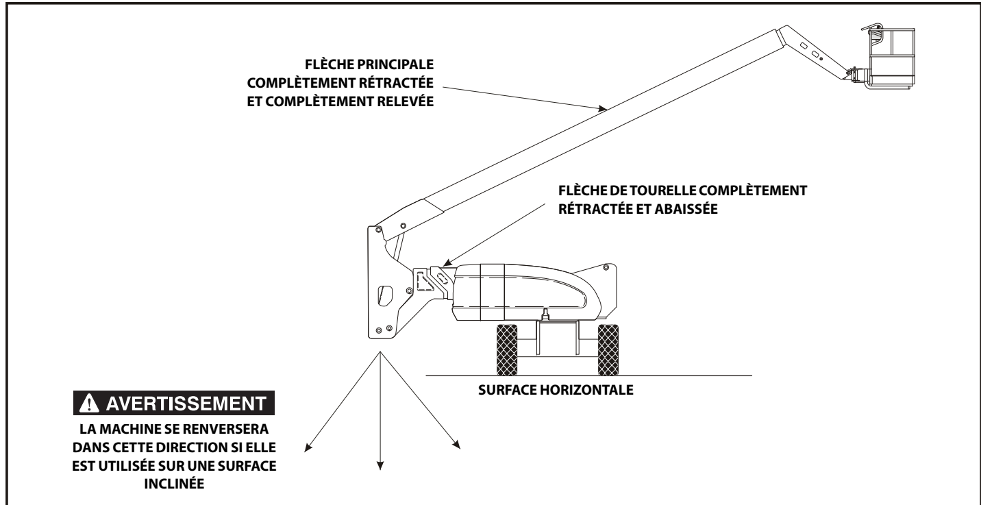
Figure 4-2. Positions les moins stables vers l'arrière (fiche 1 sur 2)
