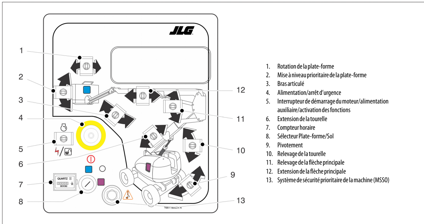
Figure 3-2. Console de commande au sol avec système de sécurité prioritaire de la machine (MSSO) (CE uniquement)
