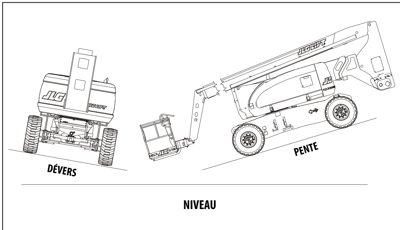
Figure 4-4. Pente et dévers
