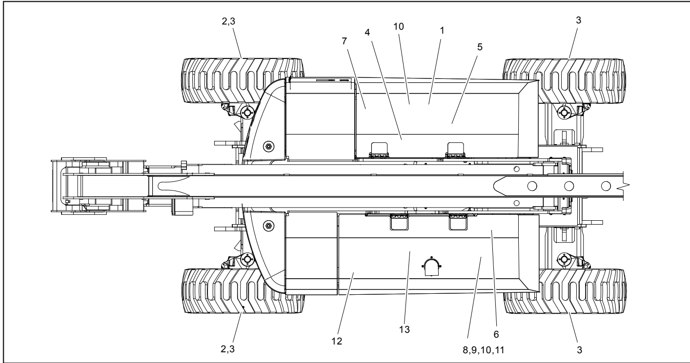
Figure 6-5. Schéma de lubrification et de maintenance
