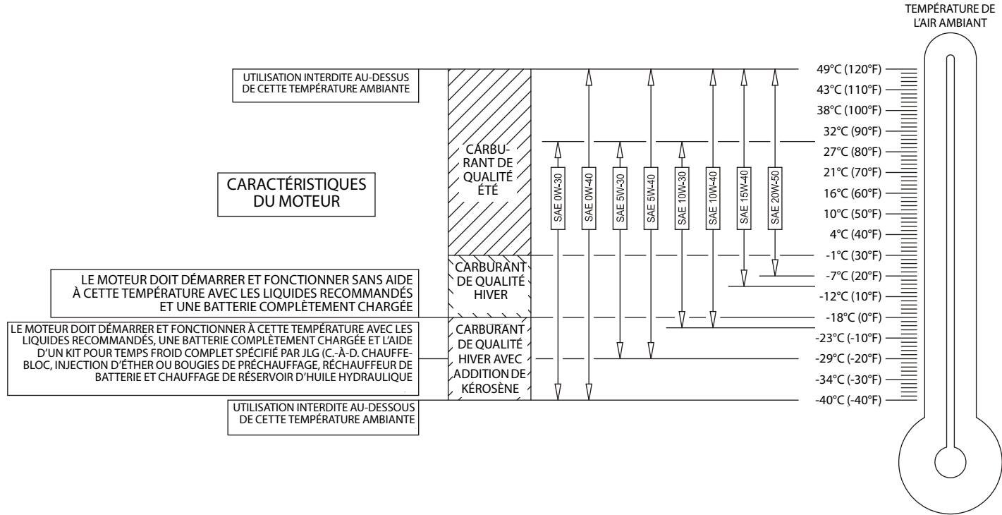
Figure 6-1. Spécifications de température de fonctionnement du moteur — Deutz — Fiche 1 sur 2
