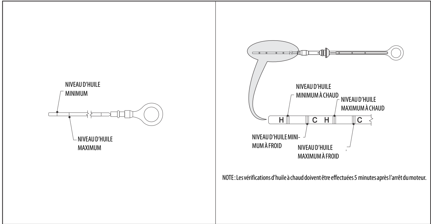
Figure 6-6. Jauge d'huile de moteur Deutz 2011
