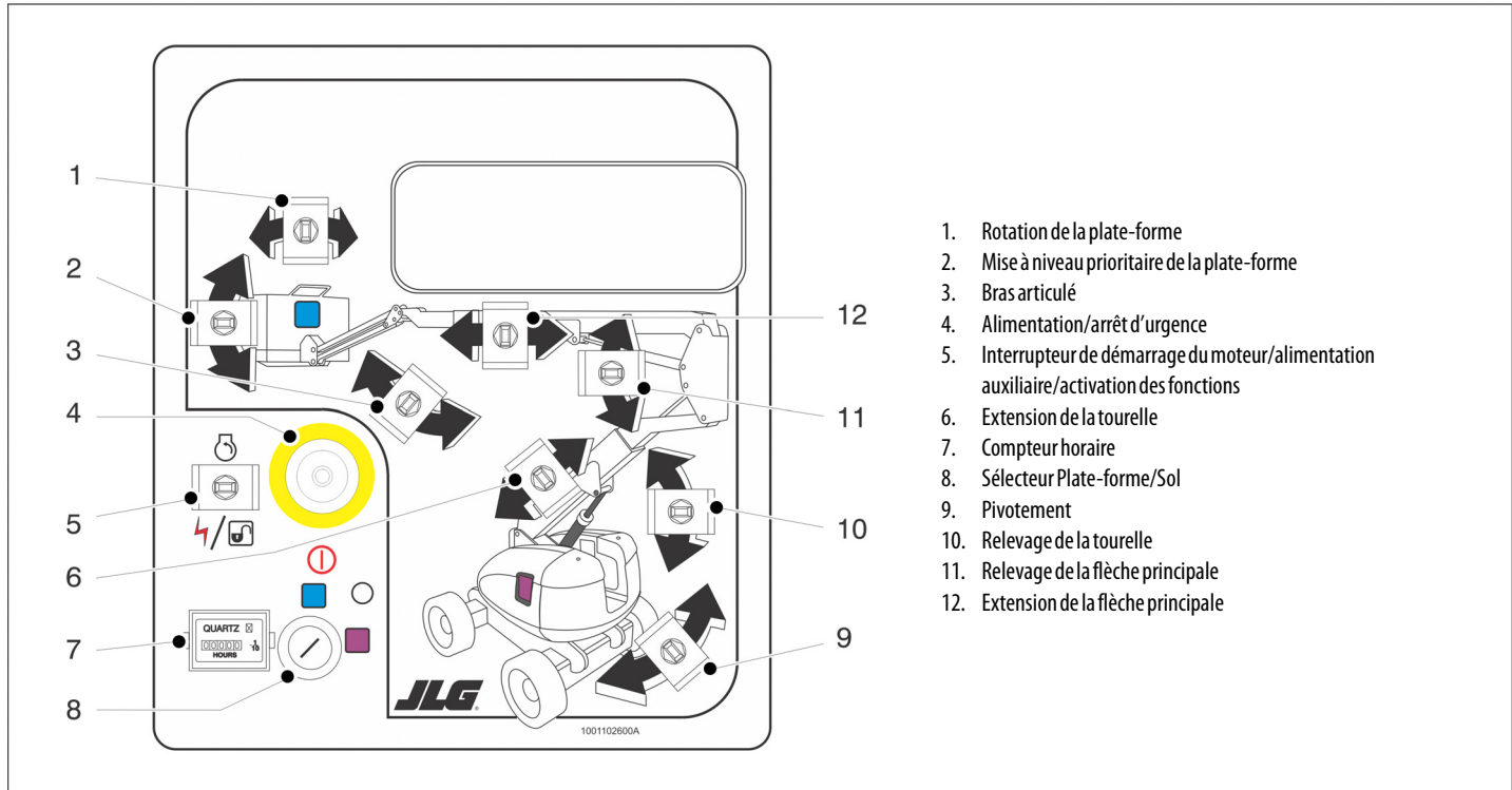
Figure 3-1. Console de commande au sol
